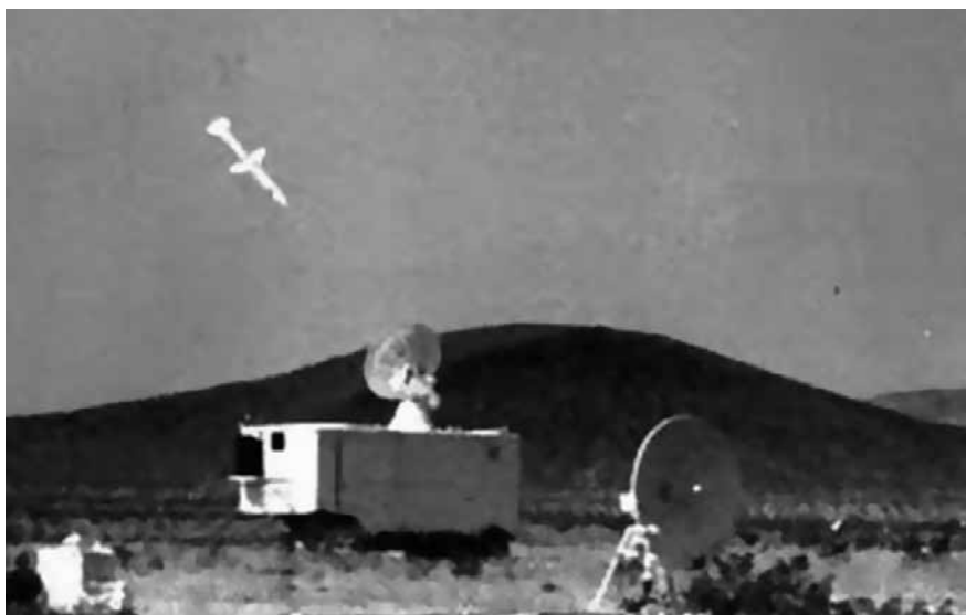
Tên lửa Shrike tiêu diệt một đài radar trong thử nghiệm
